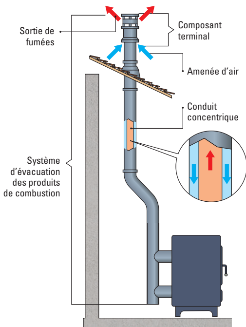
Exemple d'un poêle à granulés raccordé sur système d'évacuation des produits de combustion — zone 1 et 2
