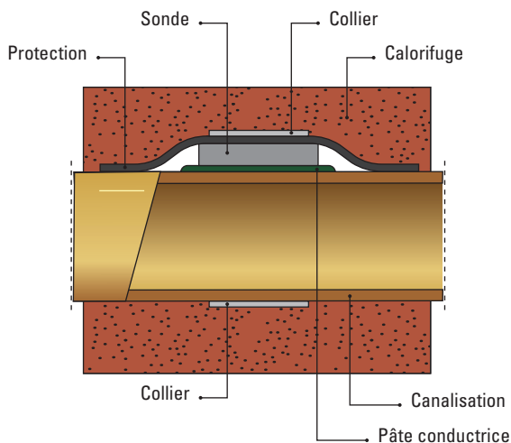
Exemple de pose d'une sonde d'applique
